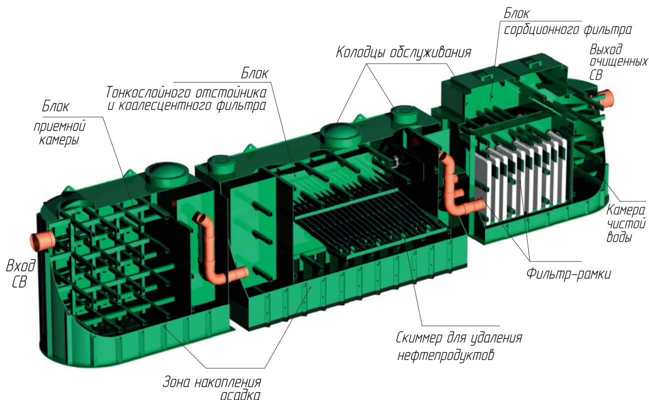
Рисунок 6. Устройство Станции Alta Rain Pro 50 – 150
